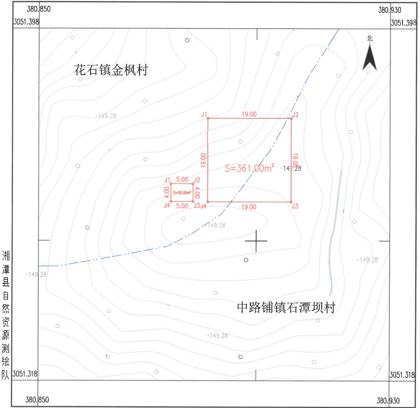
湘潭县白石镇分散式风电场建设项目勘测定界图(3#)
