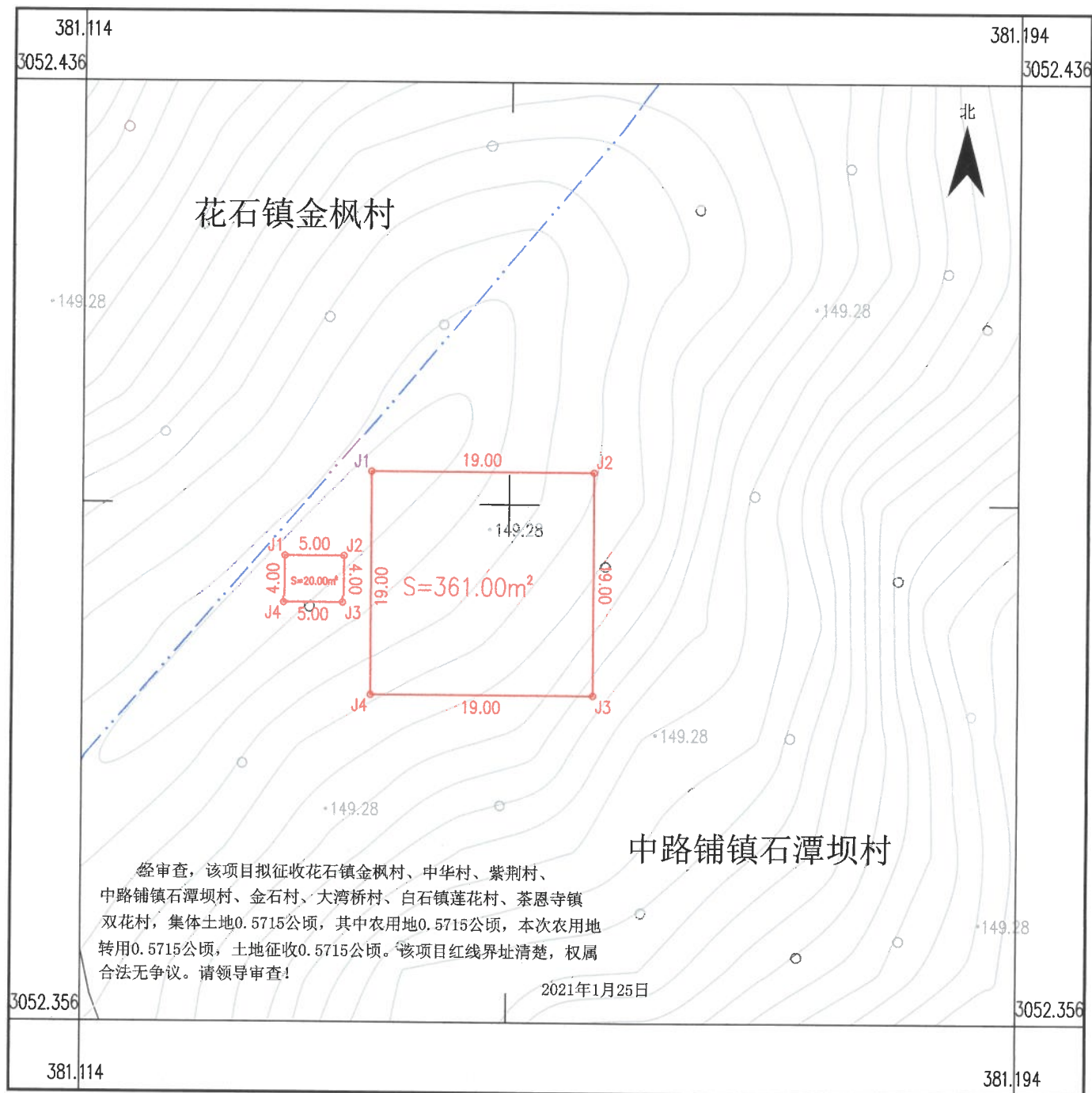
湘潭县白石镇分散式风电场建设项目勘测定界图(2#)
