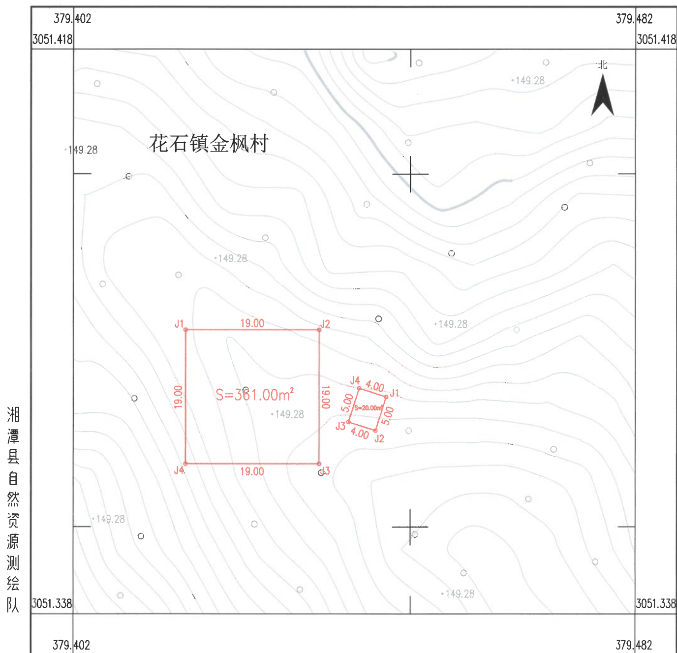
湘潭县白石镇分散式风电场建设项目勘测定界图(7#)
