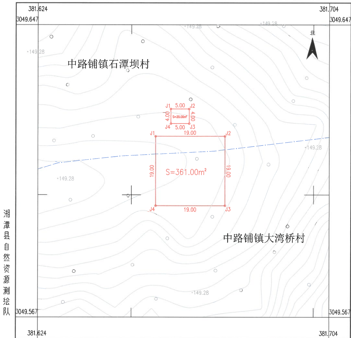
湘潭县白石镇分散式风电场建设项目勘测定界图(9#)
