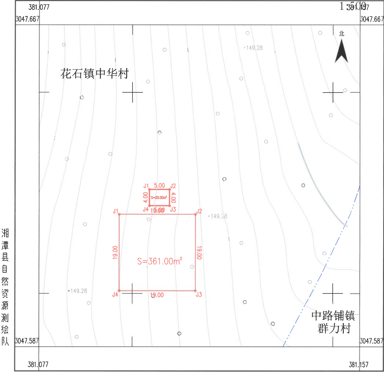
湘潭县白石镇分散式风电场建设项目勘测定界图(10#)
