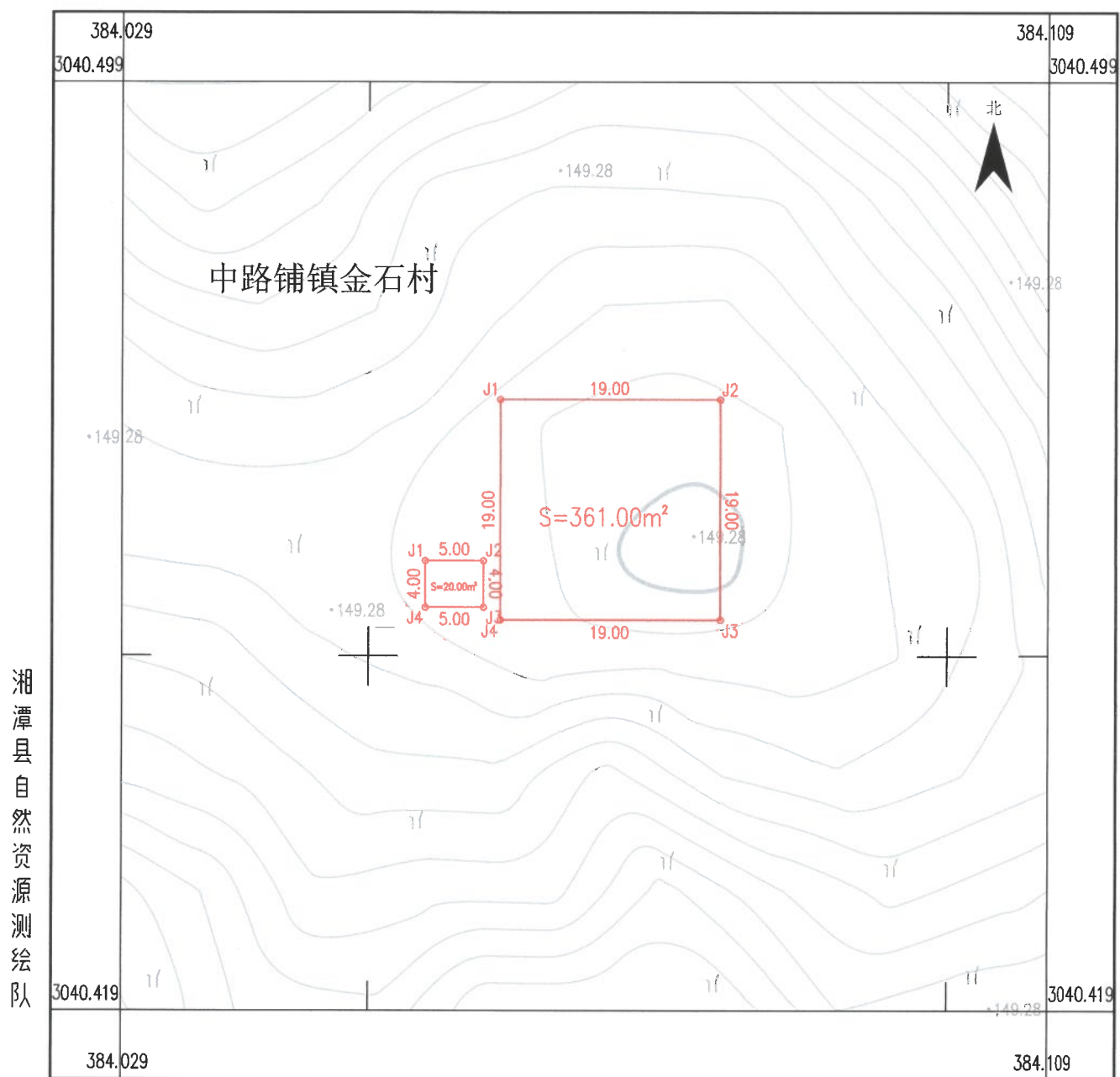
湘潭县白石镇分散式风电场建设项目勘测定界图(12#)
