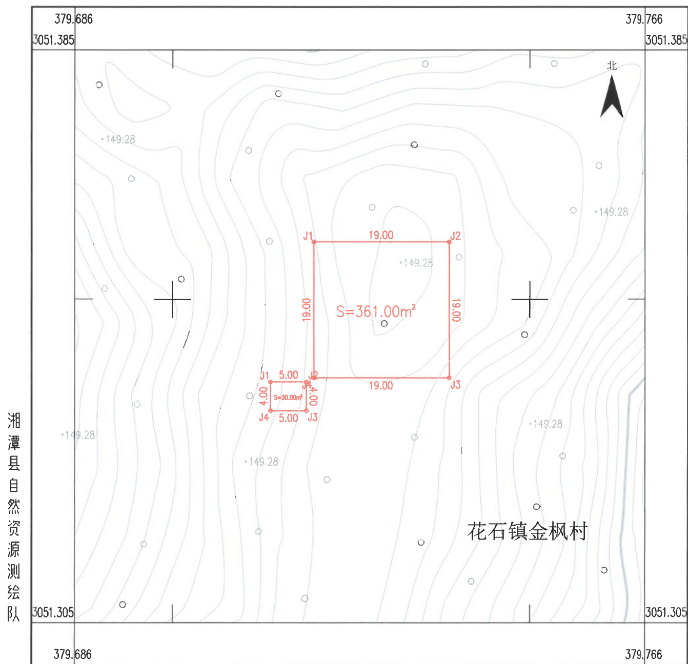
湘潭县白石镇分散式风电场建设项目勘测定界图(6#)
