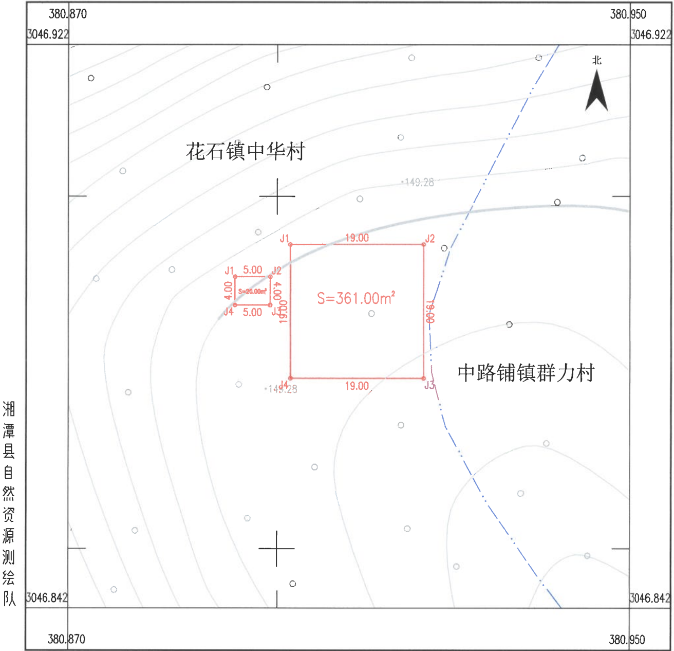
湘潭县白石镇分散式风电场建设项目勘测定界图(11#)
